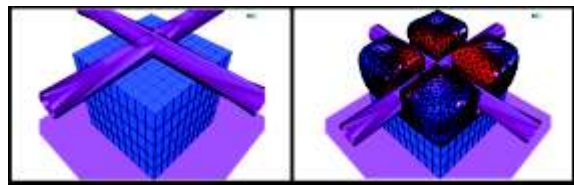
三维实体网格重划分实例
