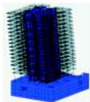
建筑结构连续坍塌模拟
